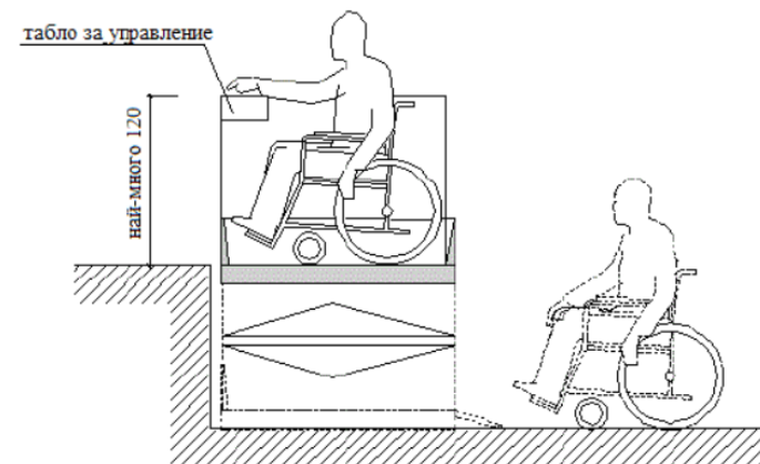
Фиг. 29. Подемни платформи
